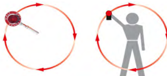
Abbildung 14 – Anhalten eines Zuges (Notmaßnahme)
