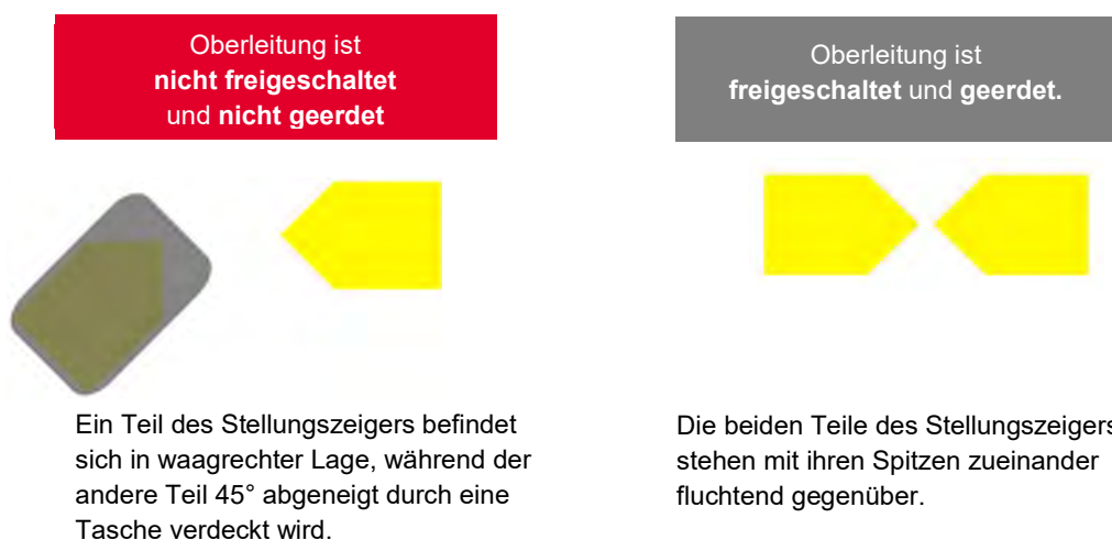
Abbildung 47 – Stellscheibe
