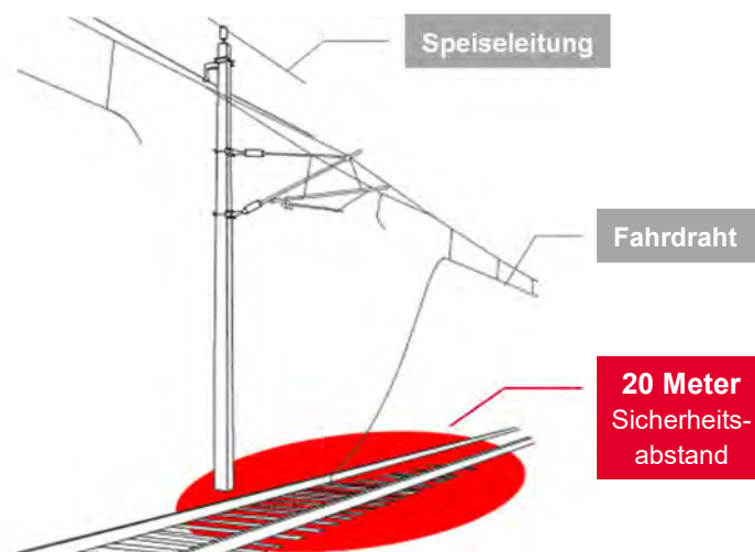
Abbildung 26 – Oberleitungsanlage
