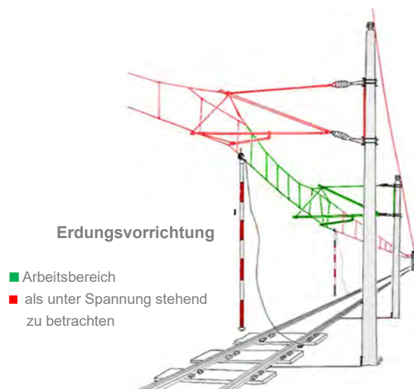
Abbildung 21 – Oberleitungsanlage
