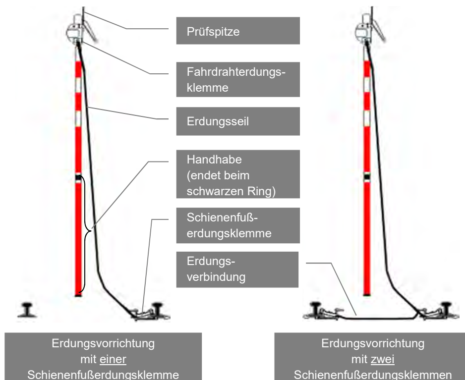
Abbildung 54 – Erdungsvorrichtung, Beschreibung
