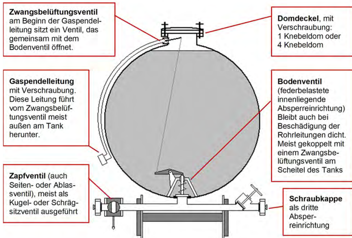
Abbildung 65 - Aufbau Kesselwagen
